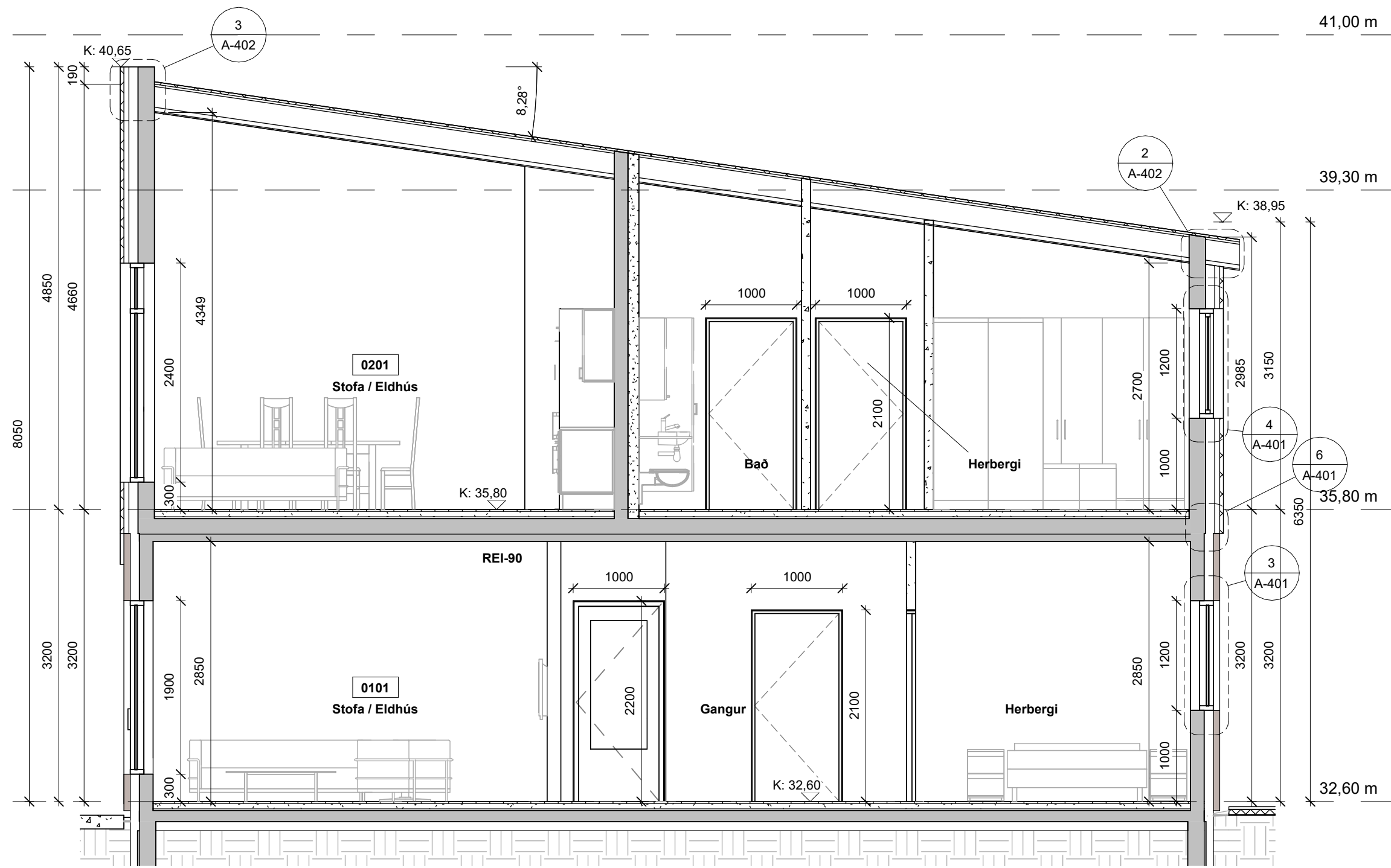
- SNID B 1 : 50
