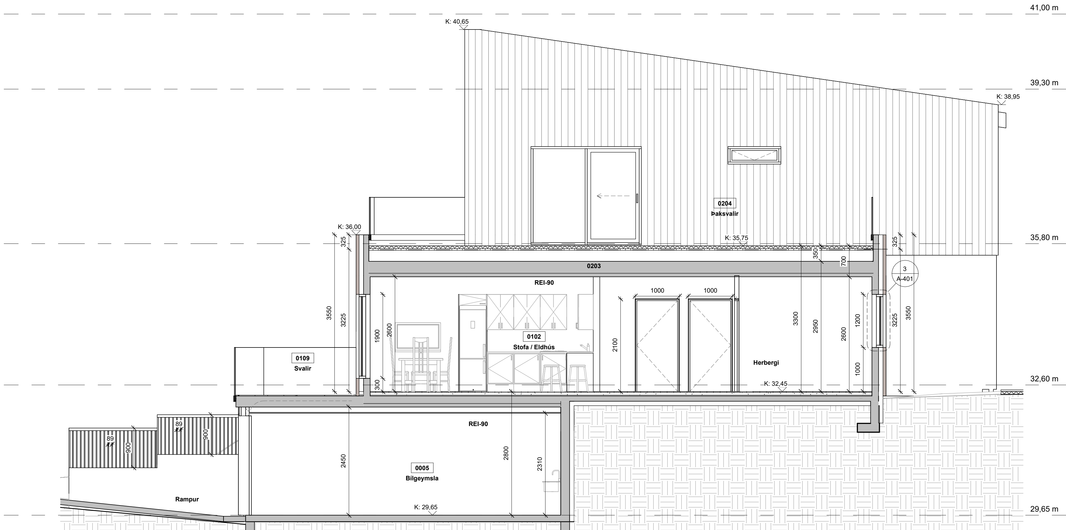
- SNID C 1 : 50
