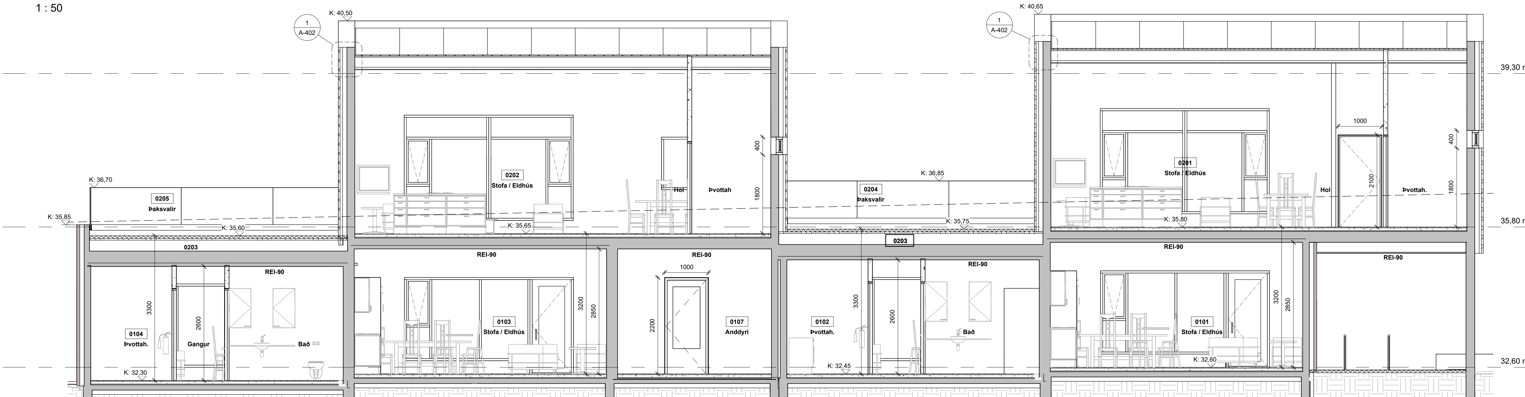
- SNID H 1 : 50
