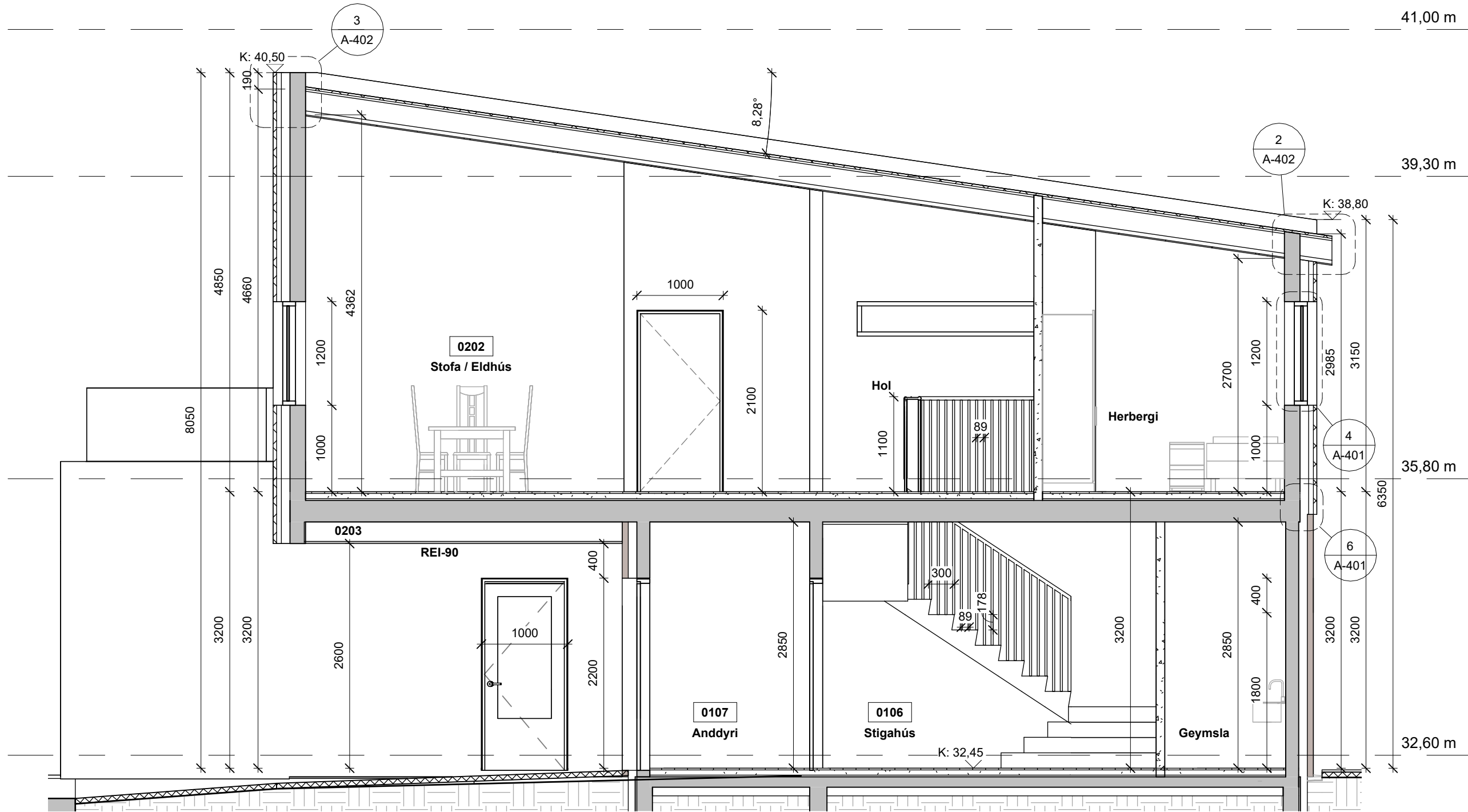
- SNID D 1 : 50
