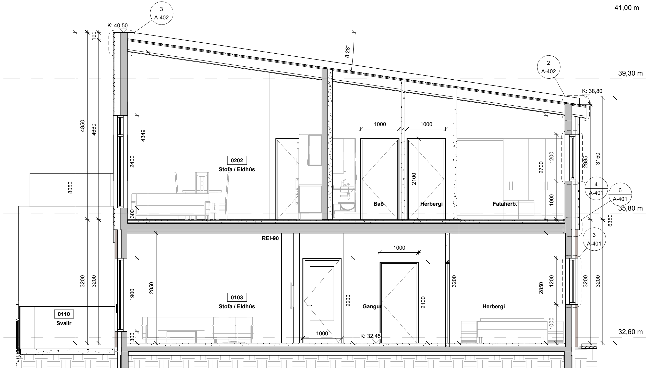
- SNID E 1 : 50
